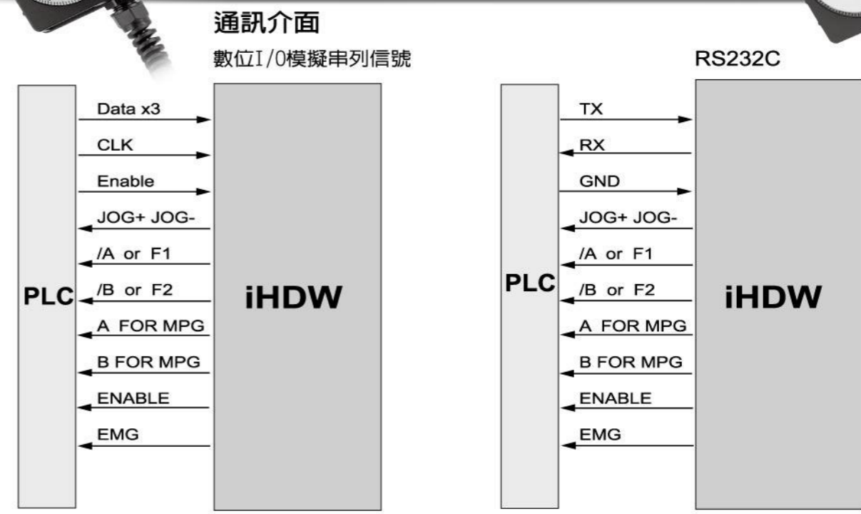
顯示型接線方塊圖：
