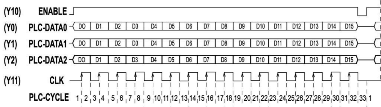
顯示型資料傳輸時序圖 (數位I/O模擬串列信號)：
